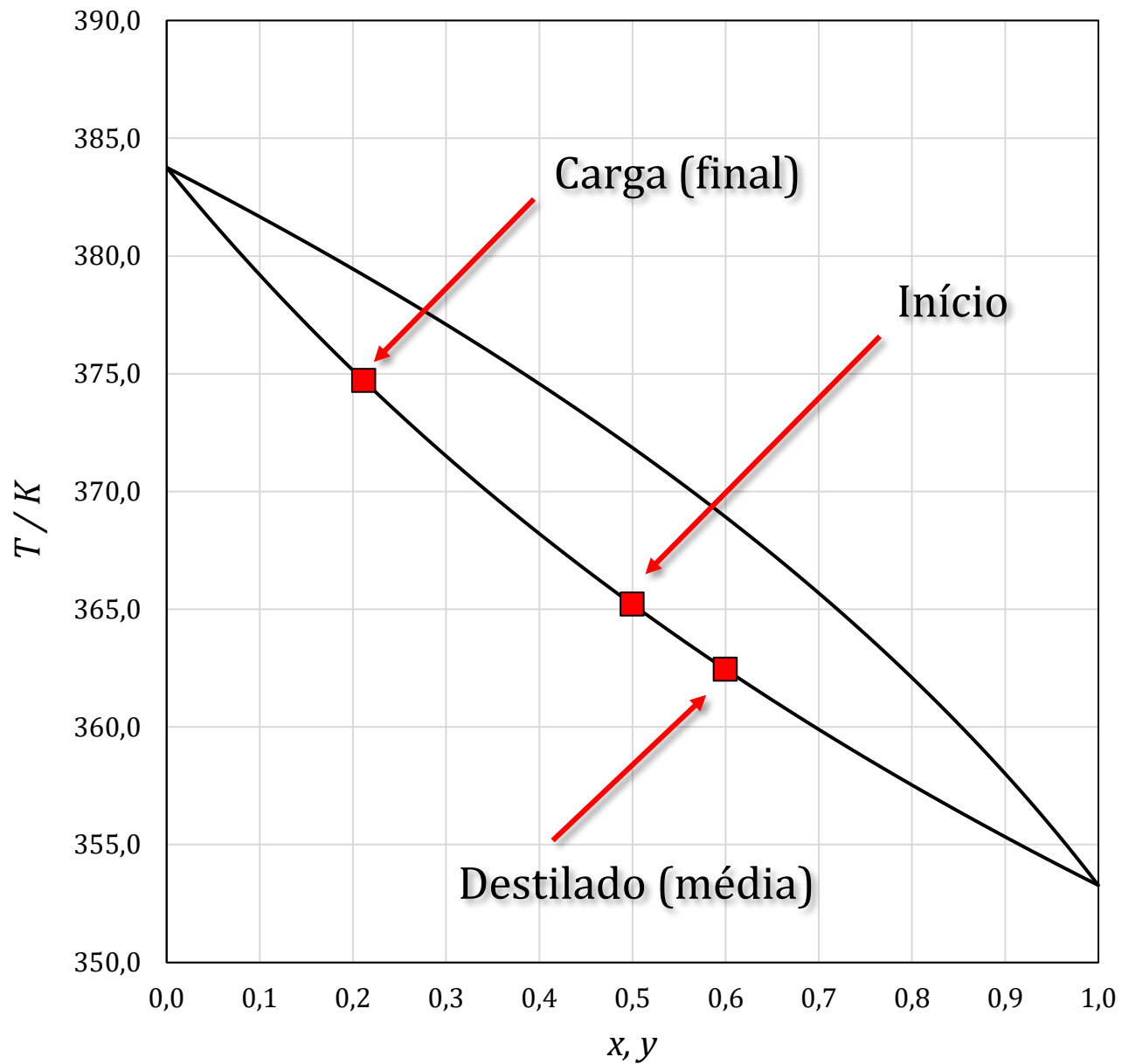
Diagrama Txy da mistura benzeno / tolueno a 101,3 kPa
