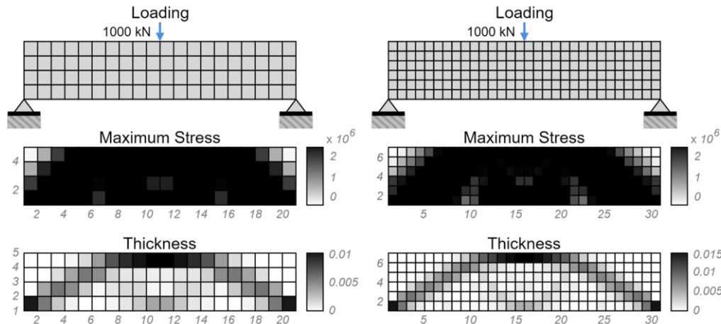
Figura 7 - Placa biapojada com carregamento concentrado
