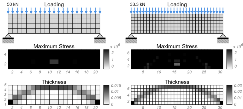
Figura 6 - Placa biapoada com carregamento uniforme
