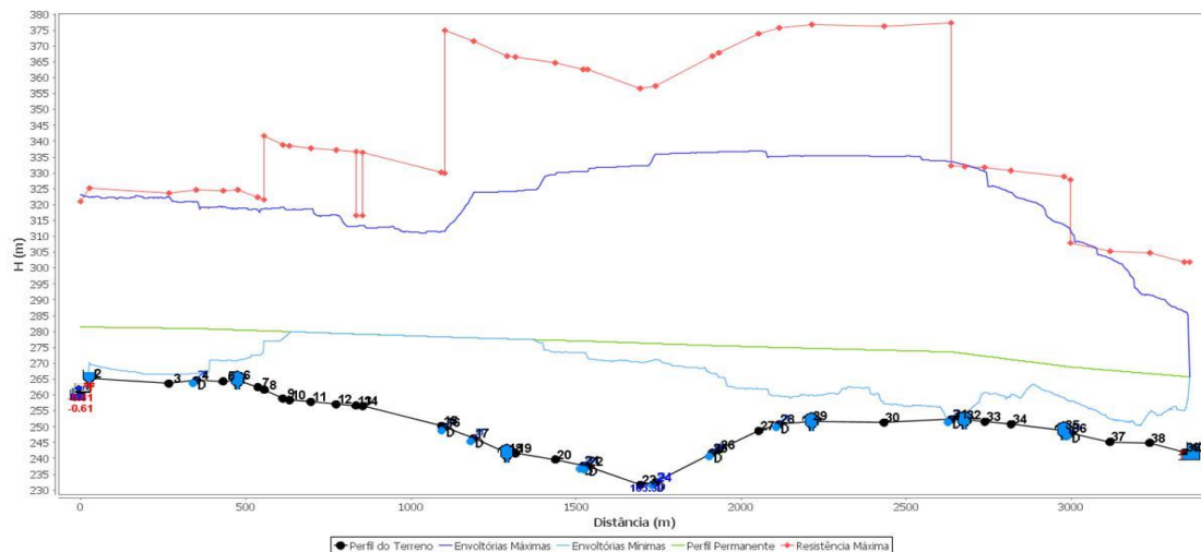
Figura 22. Solução única. Troca de tubos (Classes de Pressão) + 1 TAU + 5 Ventosas.
