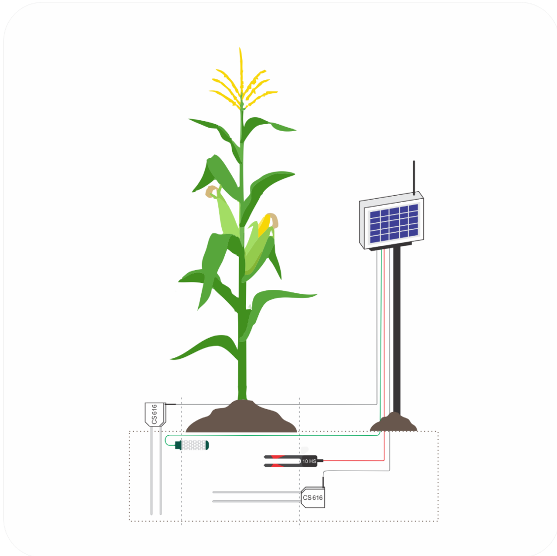
Figura 4. Diferentes tipos de sensores utilizados na medição do conteúdo e do potencial de água no solo e a posição do sensor, em manejo da irrigação de culturas anuais. Modelo CS616 (Campbel Sci., Inc) e 10 HS (Decagon) são sensores tipo FDR, e o watermak (verde) é um sensor de resistência elétrica (Irrrometer).
