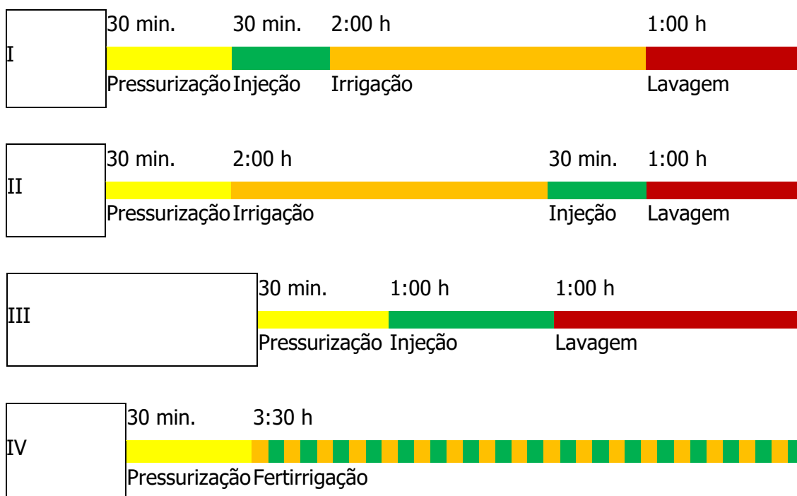
Figura 2. Cenários de fertirrigação, considerando o tempo de avanço de 1 hora, para aplicação de nutrientes em solo.
