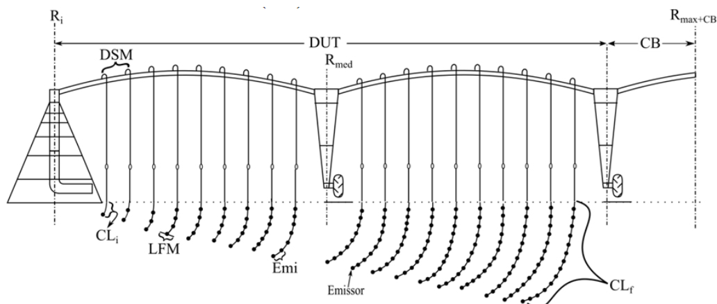
Figura 3. Esquema de um sistema de irrigação por gotejamento móvel em pivô central (PMDI - Pivot Mobile Drip Irrigation ). R_i - raio inicial; R_{med} - raio médio do pivô; R_{max+CB} - raio máximo do pivô com balanço; DUT - Distância até a última torre; CB - comprimento do balanço; DSM - Distância entre saídas de mangueira; CL_i - comprimento de tubo gotejador da primeira linha; CL_f - comprimento de tubo gotejador da última linha; LFM - largura da faixa molhada do emissor; Em_i - espaçamento entre emissores no tubo gotejador (ALMEIDA et al. , 2017).
