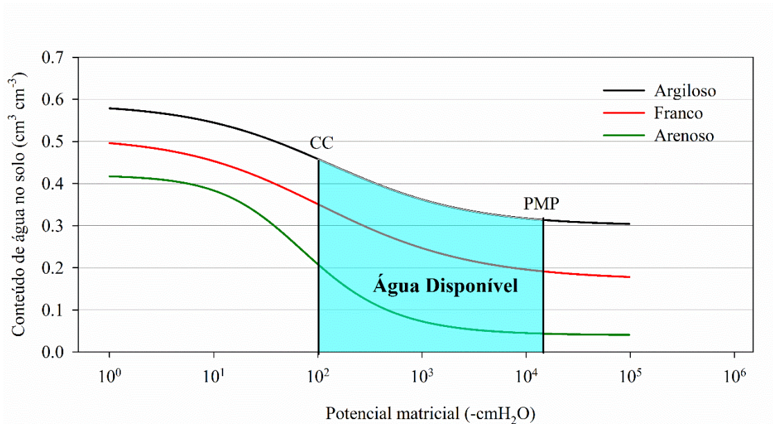
Figura 1. Curvas de retenção de água para solos de textura argilosa, franca e arenosa, da umidade de saturação ao ponto de murcha permanente. A umidade entre a capacidade de campo ( \theta_{100\text{ cm}} ) e o ponto de murcha permanente ( \theta_{15000\text{ cm}} ) corresponde a água disponível (área hachurada em azul claro), para as três classes de textura de solo.
