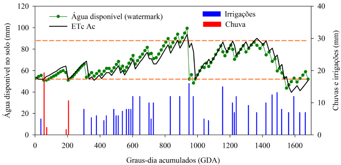
Figura 8. Balanço hídrico combinado (status de água no solo + ETc) para a determinação do momento de irrigar na cultura do milho A ETc (estimada através da metodologia ETc-Kc) e sensores de umidade tipo Watermark são combinados para melhorar a gestão da irrigação.
