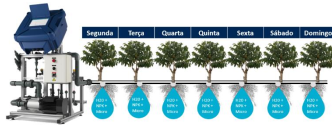
Figura 17. Vista de um sistema de fertirrigação automático denominado de nutr irrigação com aplicações diárias de nutrientes.
