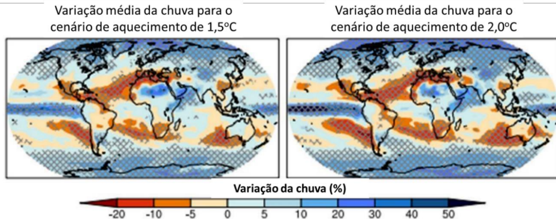
Figura 8. Cenários de mudanças climáticas (chuva) para 2100, considerando-se os cenários de aumento da temperatura de 1°C e 2°C, onde observa-se redução de chuvas em grande parte do Brasil (INTERGOVERNAMENTAL PANEL CLIMATE CHANGE, 2014).
