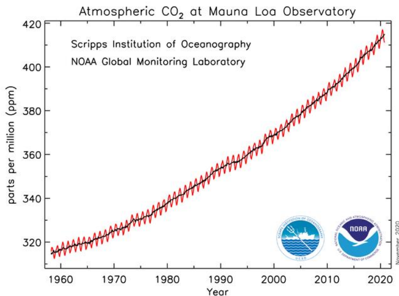
Figura 6. Variação temporal da concentração de CO 2 atmosférico observado na ilha de Mauna Loa, Havaí, Estado Unidos, desde o final dos anos 50 (EARTH SYSTEM RESEARCH LABORATORY, 2020).
