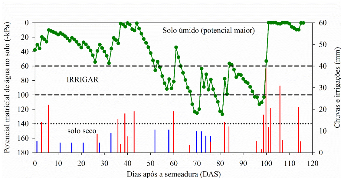
Figura 3. Flutuação do potencial matricial de água no solo (-kPa) durante uma estação de cultivo de milho, com sensores Watermark instalados a 10, 30 e 50 cm de profundidade, em área irrigada por pivô central. Barras em azul e vermelho representam as irrigações e precipitações pluviais. As linhas tracejadas (---), referem-se ao limite de potencial considerado como críticos para o início das irrigações, e (....) solo extremamente seco.
