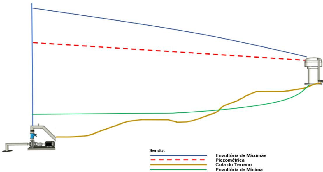
Figura 4. Representação gráfica clássica de onda de pressão: (i) elevatória (EB) em operação normal, com a pressão nos pontos representada pela linha piezométrica (vermelha tracejada); (ii) após parada súbita da EB, o líquido continua a fluir por determinado tempo, causando em primeiro lugar uma onda de sub-pressão (ou depressão, abaixo do valor da piezométrica naquele ponto); e (iii) após a onda de sub-pressão, ocorre outra de sobrepressão, e assim sucessivamente até a parada total do sistema.
