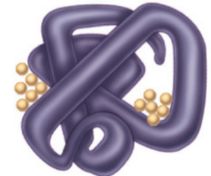
(d) Blocked Active Site
