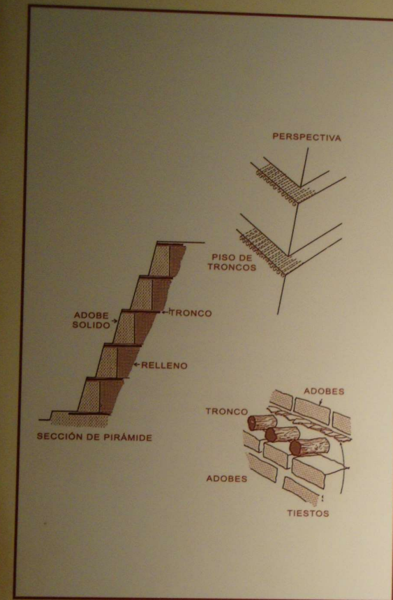
Detalle arquitectónico de la pirámide, representando la técnica de construcción del perfil escalonado.
