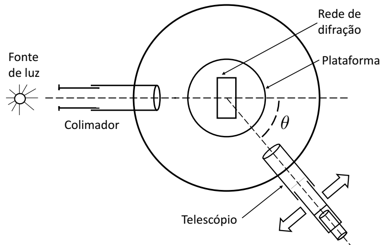
(a) Vista superior do espectroscópio óptico. Na figura é possível identificar a fonte de luz, o colimador, a rede de difração montada sobre a plataforma, e o telescópio.
