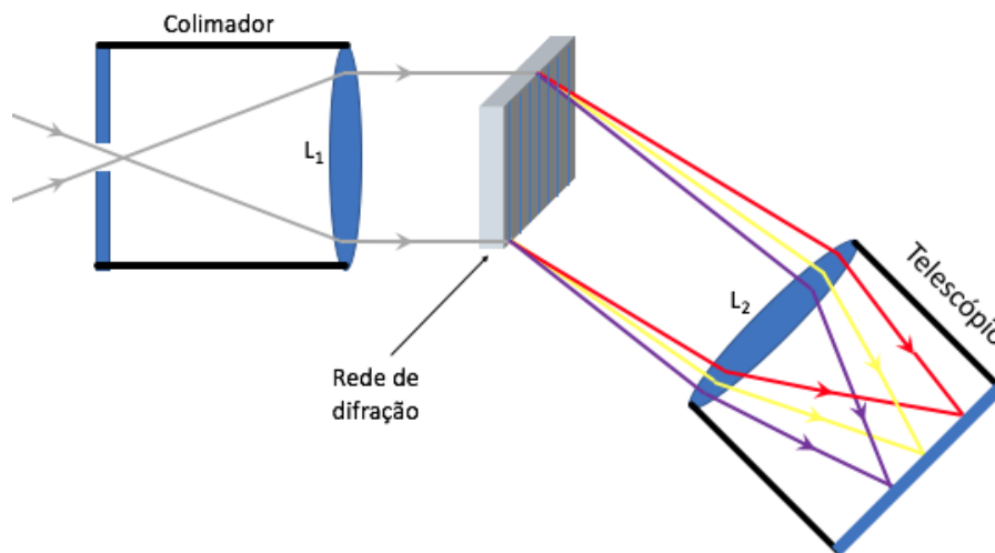
(b) Caminho do feixe de luz ao passar pelo espectroscópio óptico.
