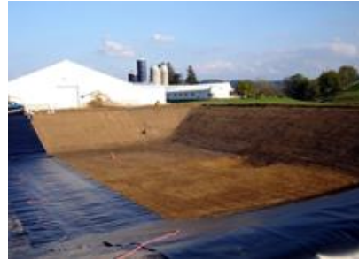
Figura 40 - Sistema de impermeabilização de base
