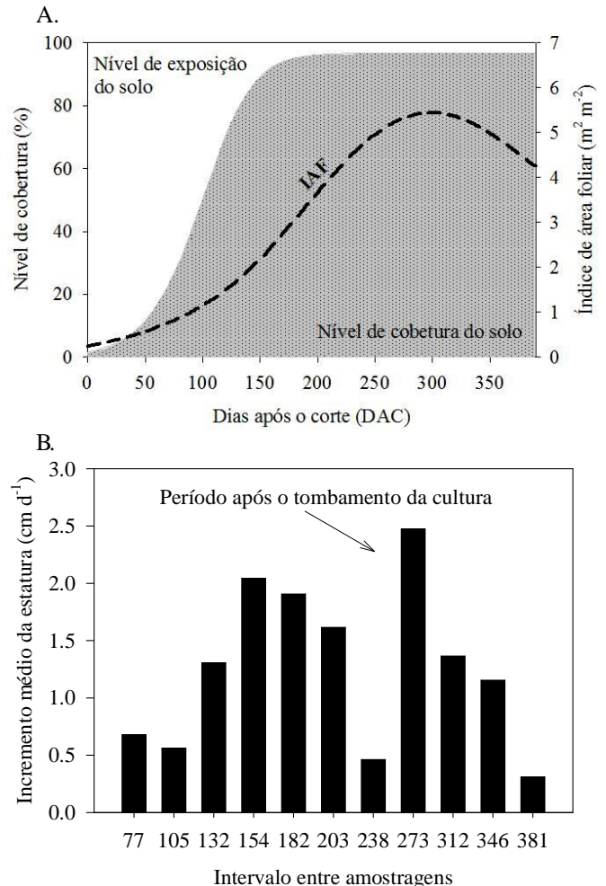
Figura 2. Nível de cobertura do solo e índice de área foliar correspondentes, em função dos dias transcorridos após o corte da cana-de-açúcar irrigada, variedade RB92579 (A). Incremento médio da estatura dos colmos durante o ciclo da cultura (B)
