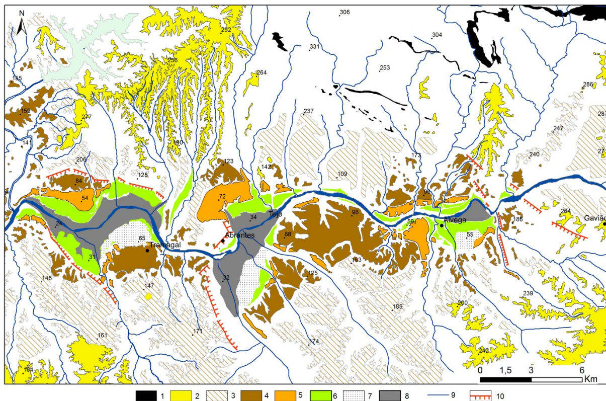
Figura 5. Mapa geomorfológico do trecho III do Baixo Tejo. 1 - crista de quartzito; 2 - superfície culminante do enchimento sedimentar da Bacia Cenozóica do Baixo Tejo; 3 - nível de erosão N1; 4 - terraços superiores (T1, T2 e T3); 5 - terraço T4; 6 - terraços inferiores (T5 e T6); 7 - cobertura de areias eólicas; 8 - planície aluvial (Holocénico); 9 - curso de água; 10 - escarpa de falha.
