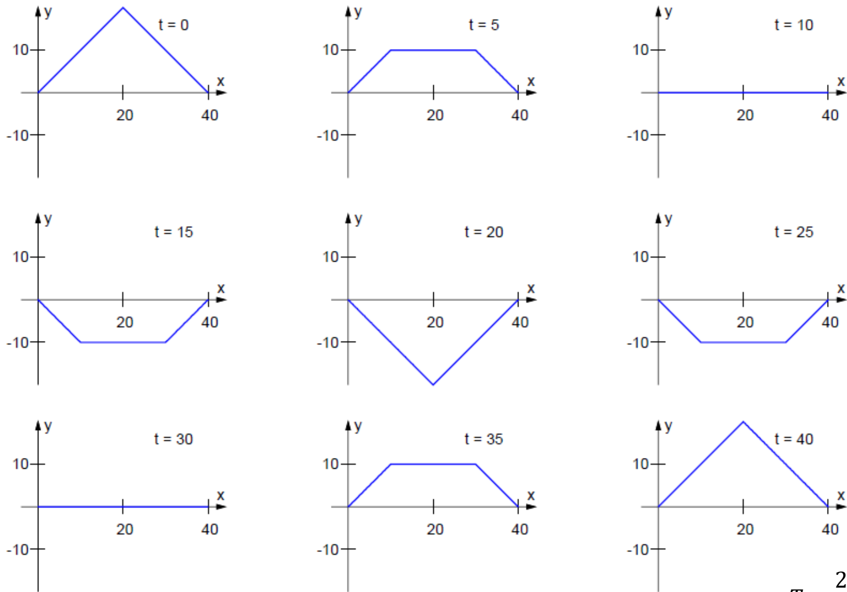
Figura 4.4 – Solução, u(x,t) , do PVIF do Exemplo 4.1.
