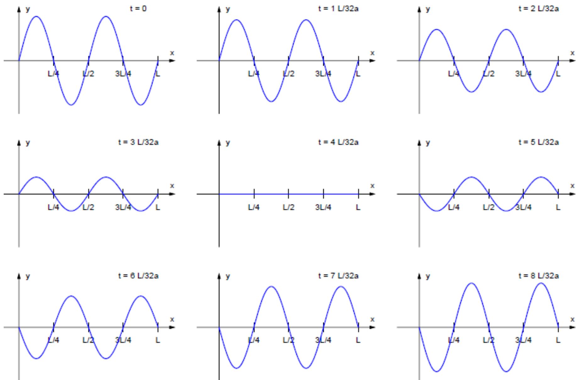
Figura 4.2 – Modo natural de vibração u_4(x, t) = \cos \frac{4a\pi t}{L} \operatorname{sen} \frac{4\pi x}{L} , para t = 0, \dots, \frac{L}{4a} .
