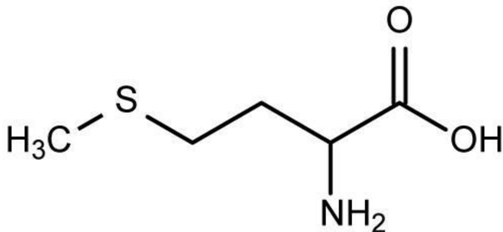
Metionina
