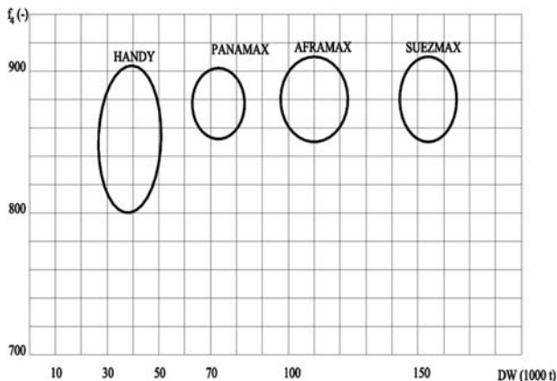
Slika 13 Faktor f_4 (tankeri)
