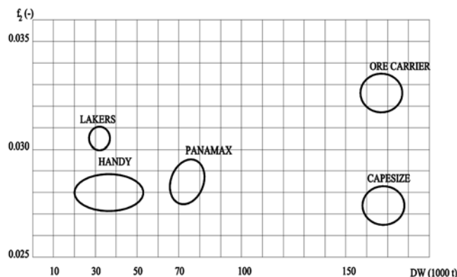
Slika 10 Faktor f_2 (brodovi za prijevoz rasutih tereta)
