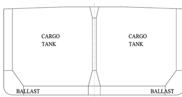
Figure 4 Typical cross-section of a product tanker Slika 4 Tipični poprečni presjek tankera za prijevoz naftnih derivata
