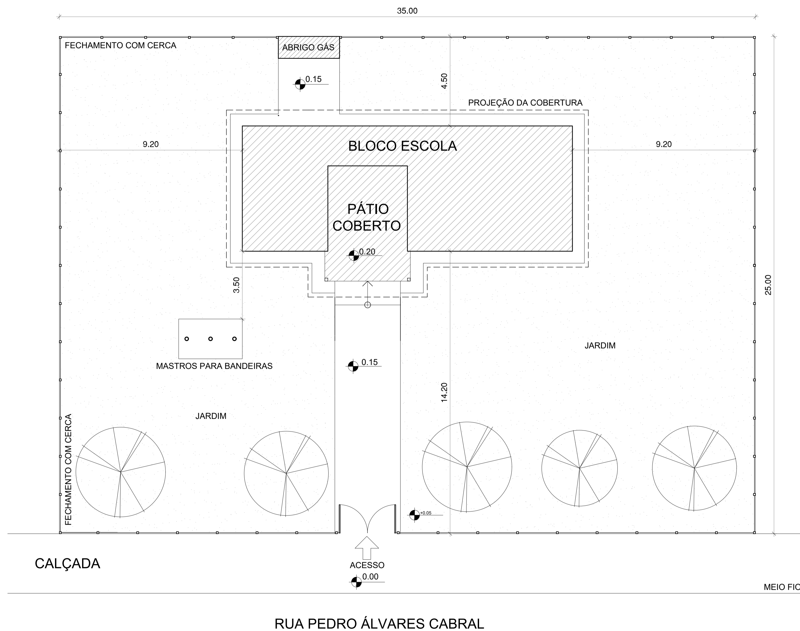
1 IMPLANTAÇÃO ESCALA 1/100
