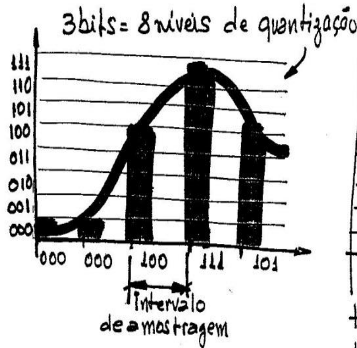
FIGURA 5- Conversor Análogo - Digital
