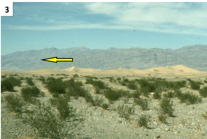
3) Duna; regime de fluxo inferior.
