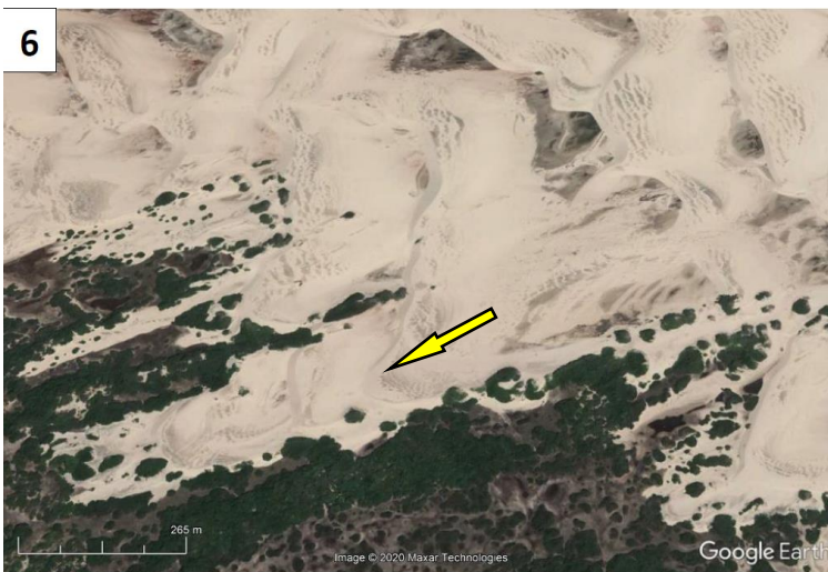
6) Duna, regime de fluxo inferior.
