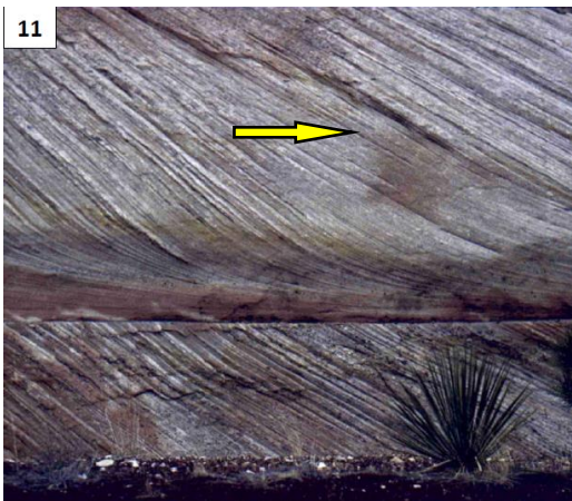
11) Estratificação cruzada, regime de fluxo inferior.
