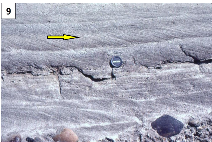
9) Estratificação cruzada, regime de fluxo inferior.
