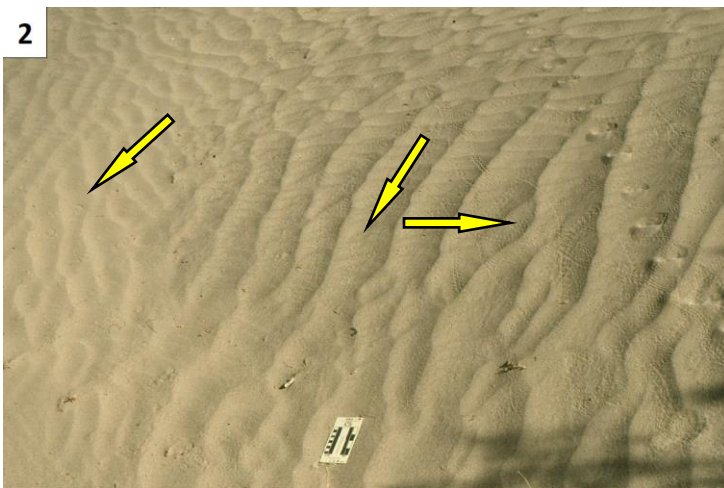
2) Marca ondulada (3 hierarquias); regime de fluxo inferior; orientação do fluxo duvidosa.
