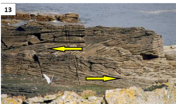
13) Estratificação cruzada; regime de fluxo superior.
