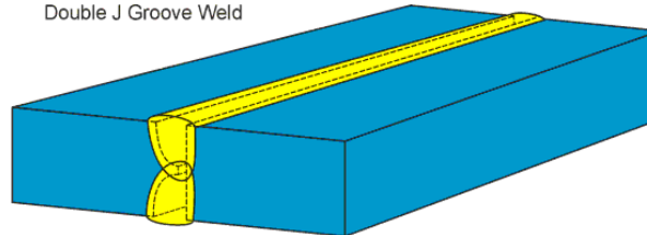
Double J Groove Weld
