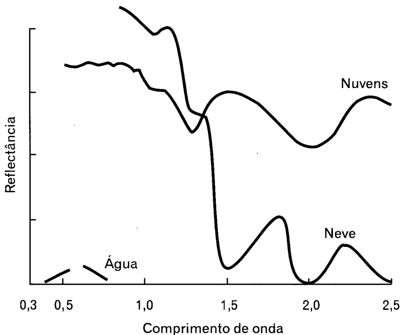
Figura 14 - Comportamento espectral da água
