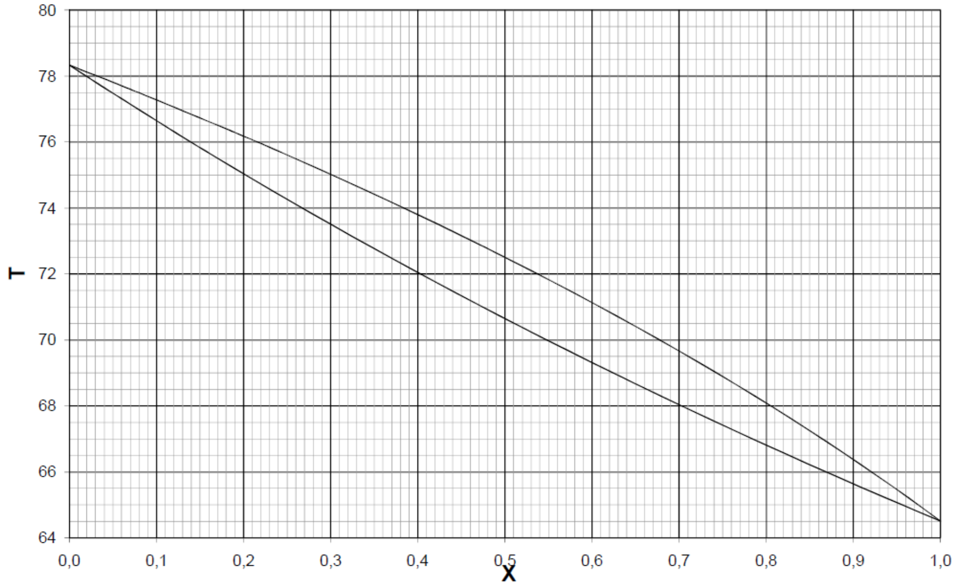
Diagrama das temperaturas de ebulição Metanol-Etanol - 760 mmHg
