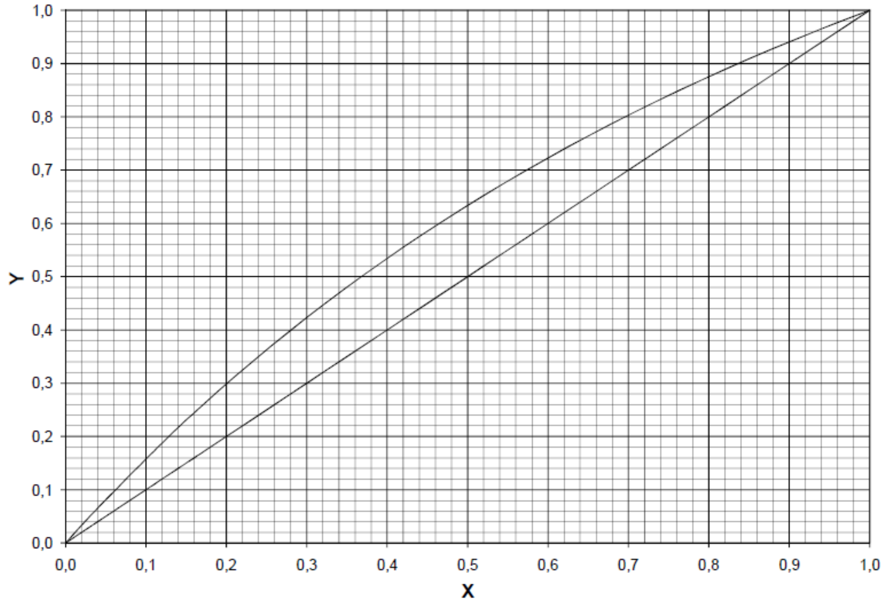
Curva de equilíbrio: Metanol-Etanol - 760 mmHg
