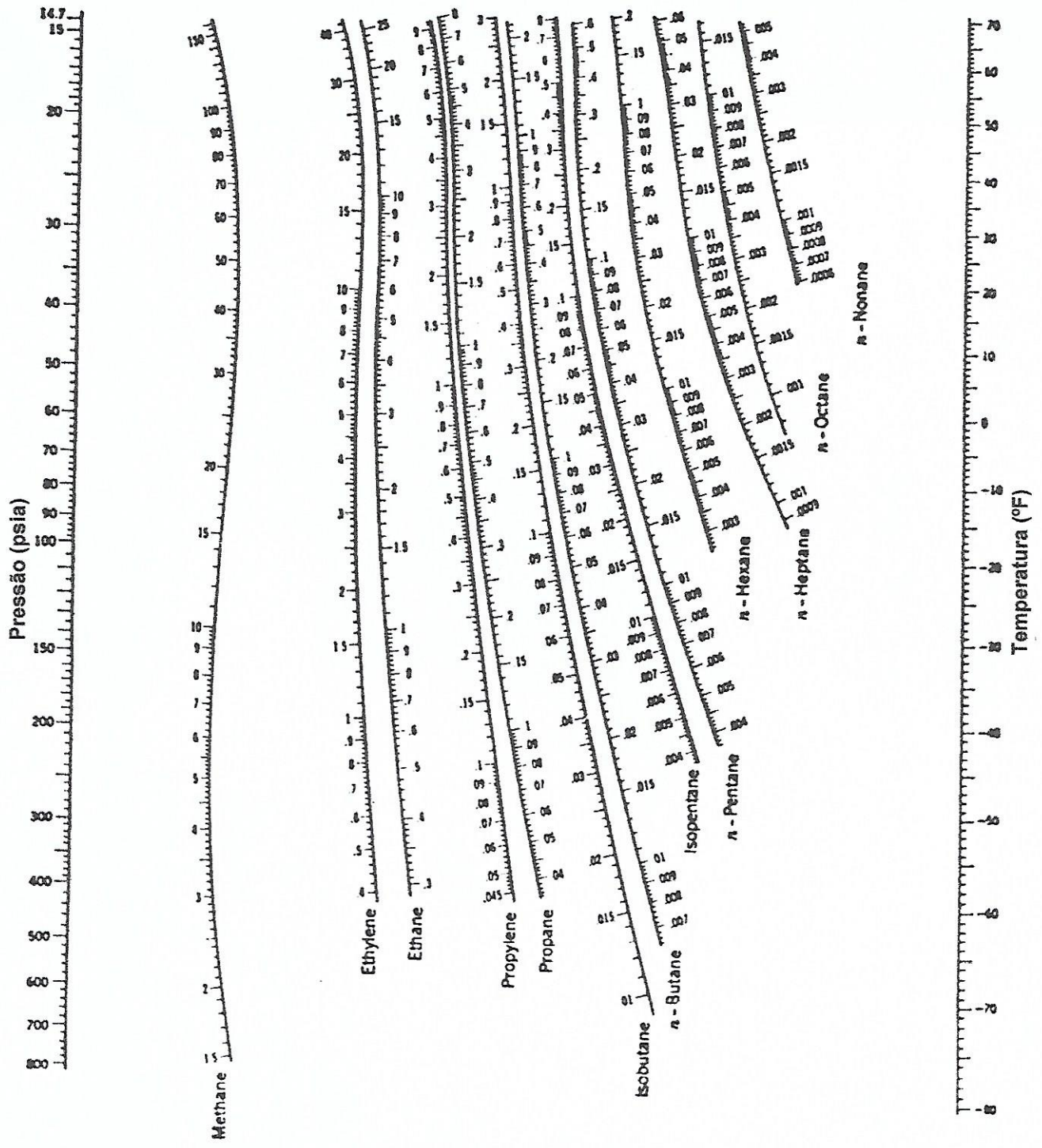
Nomógrafo de "DePriester"
