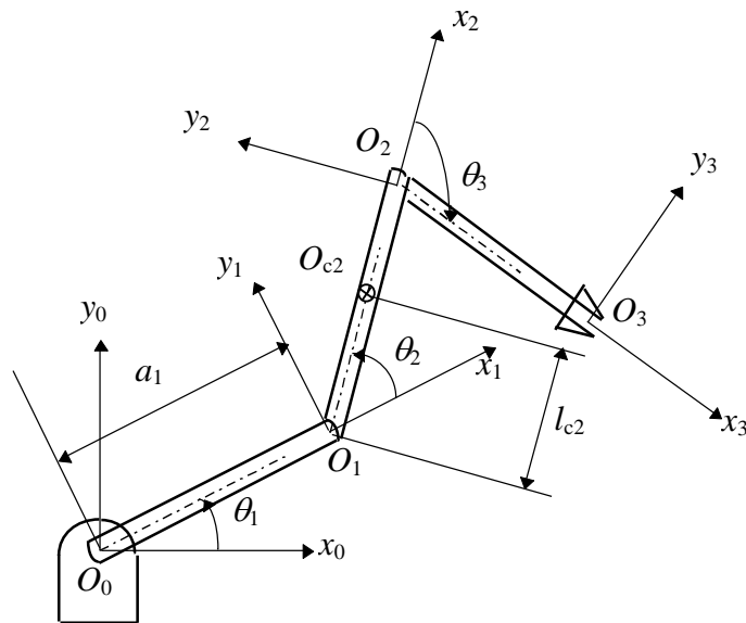
Figura 5-8: Esquema de um robô plano com três articulações de revolução.
