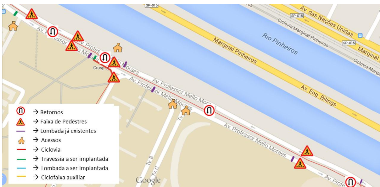
Figura 10-20 - Soluções propostas para a Av. Prof. Mello Moraes - Trecho II
