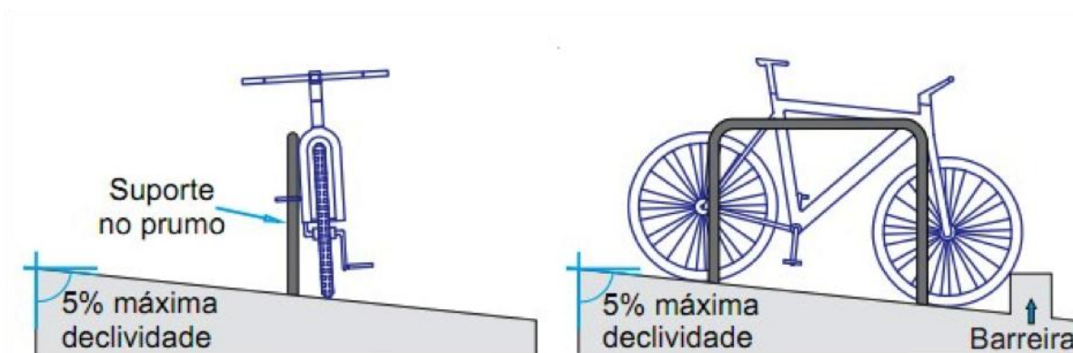
Figura 11-11 - Detalhe do modelo de suporte inglês Sheffield [127]
