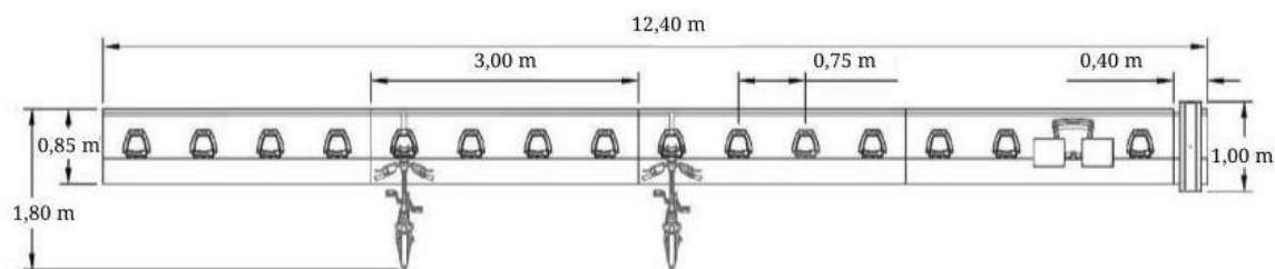
Figura 11-6 - Exemplo de dimensionamento de uma estação com 15 vagas
