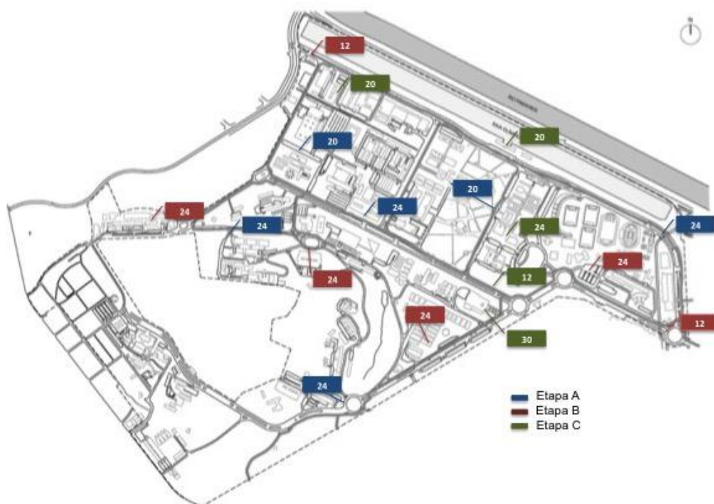
Figura 11-5 - Número de vagas de estacionamento por estação e etapa de execução final do Projeto do Sistema de compartilhamento de bicicleta na CUASO.
