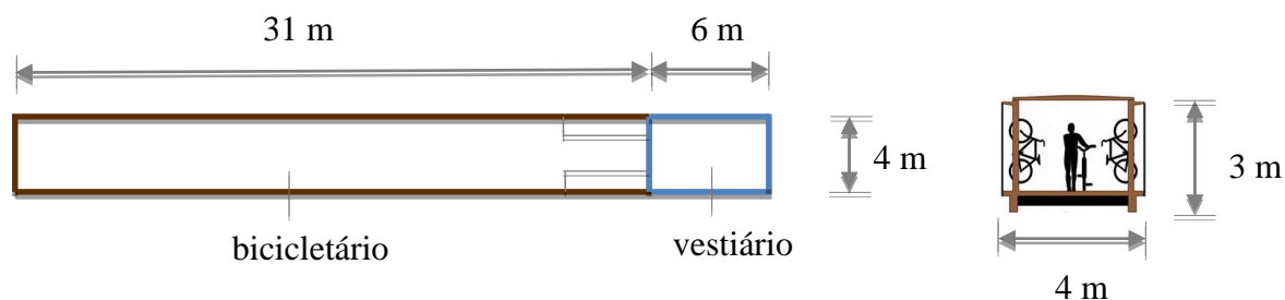
Figura 11-16 - Detalhes do bicicletário tipo A
