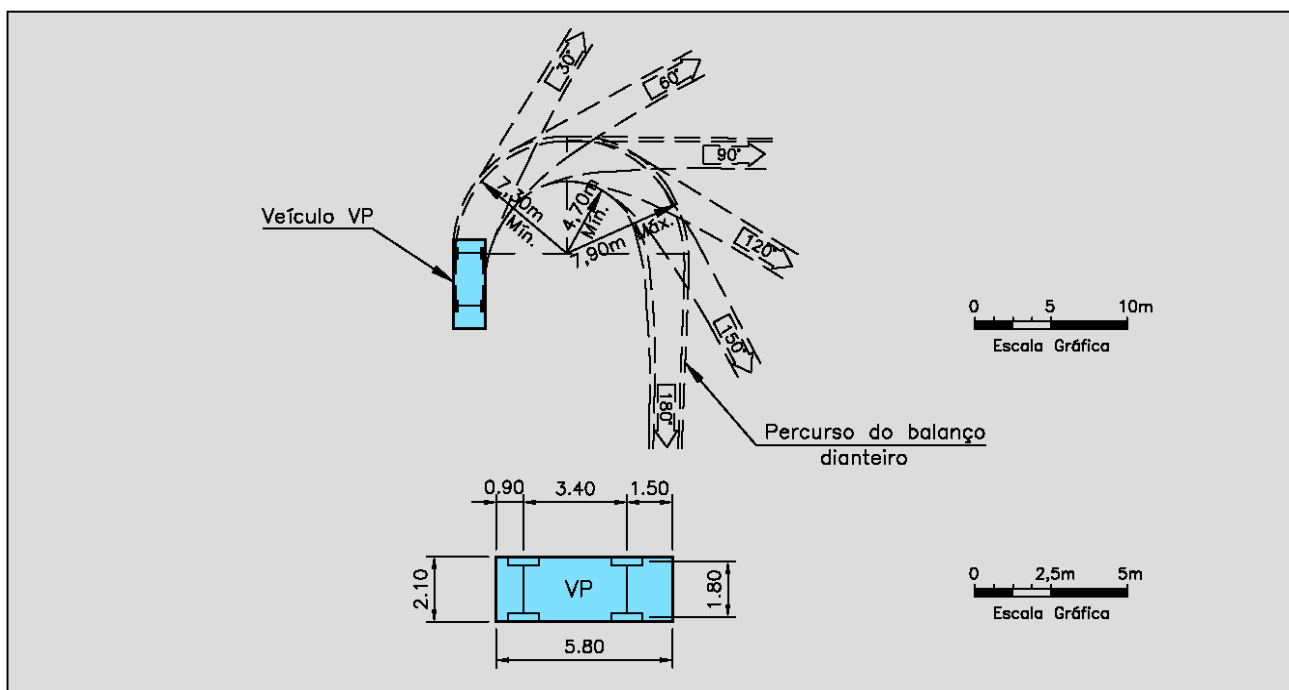
Figura 46 – Veículo de Projeto VP
