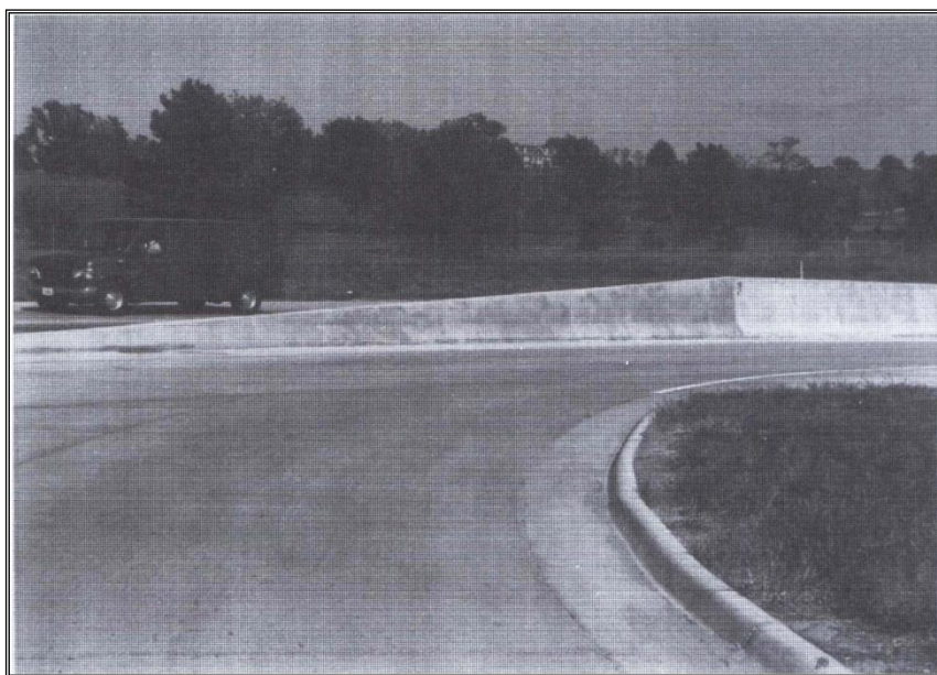
Figura 93 – Elevação gradual da crista de uma barreira de concreto
