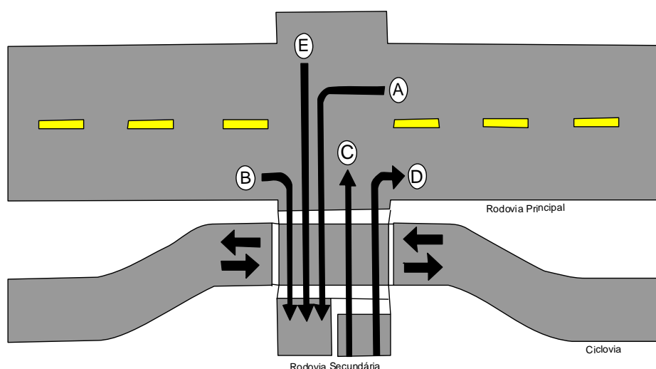
Figura 28 – Interseção de ciclovia adjacente à rodovia
