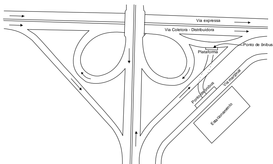
Figura 32 – Parada de ônibus em um trevo completo (□□□□□□□□)
