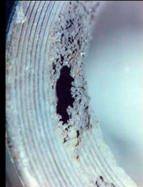
Corrosão por fresta em rosca
