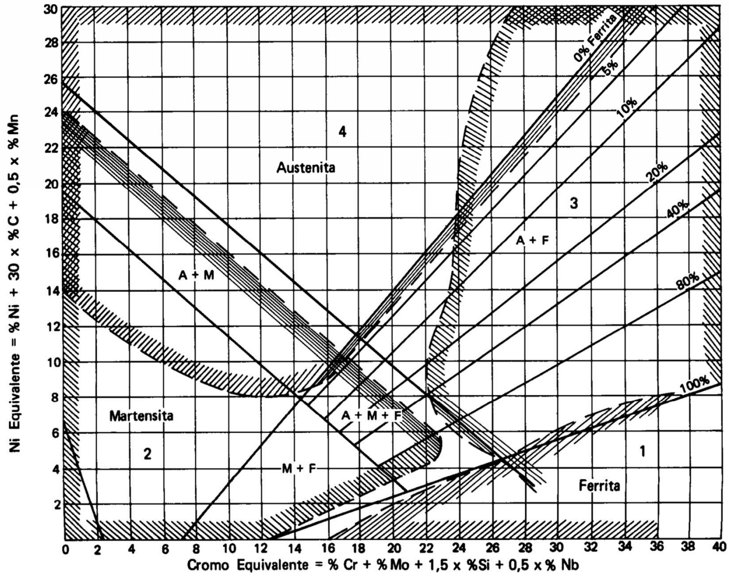
Fig. 6.28 – Diagrama de Schäffler
