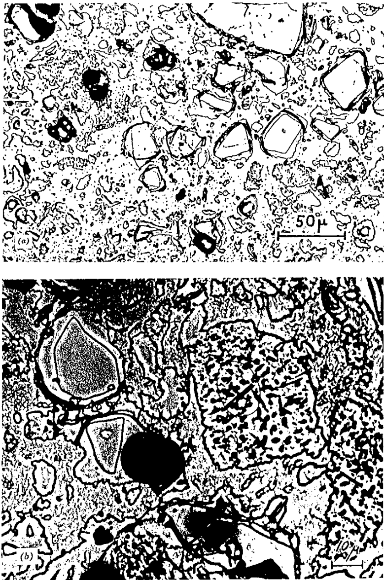
Figura 4 – Fotomicrografia de porcelana de isoladores elétricos mostrando grãos de quartzo com líquido na sua volta, grãos de feldspato com agulhas de mulita não resolvidas, matriz de argila não resolvida e poros escuros.
