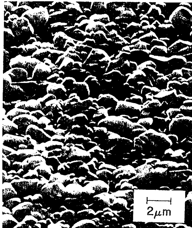
Figura 13 – Superfície da Al 2 O 3 99%, sinterizada apresentando grãos finos.
