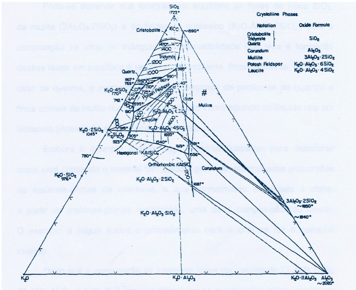
Figura 2 – Diagrama ternário K 2 O-Al 2 O 3 -SiO 2
