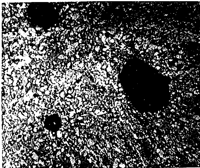
Figura 11 – Microestrutura da cerâmica enstatita.
