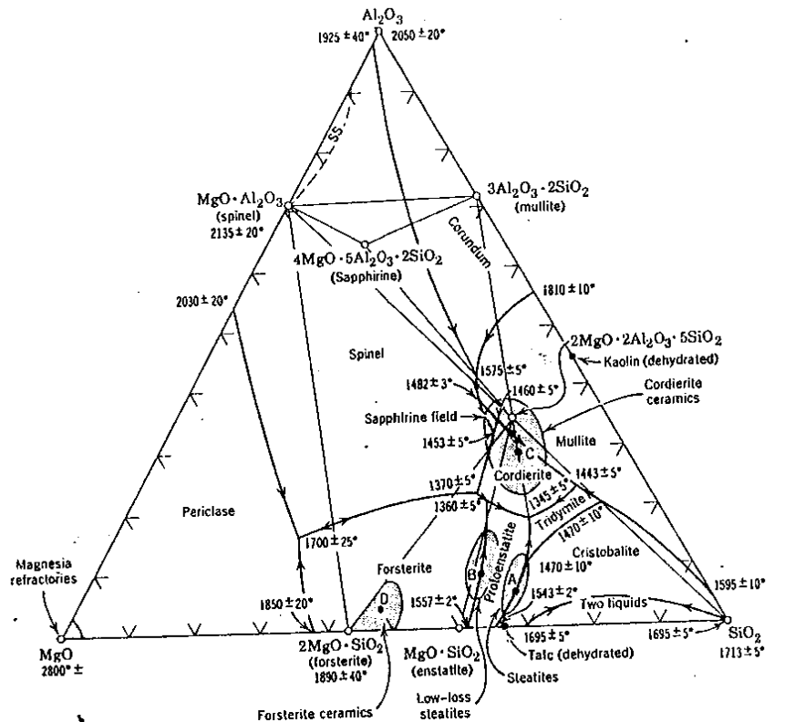
Figura 9 – Diagrama MgO-Al 2 O 3 -SiO 3
