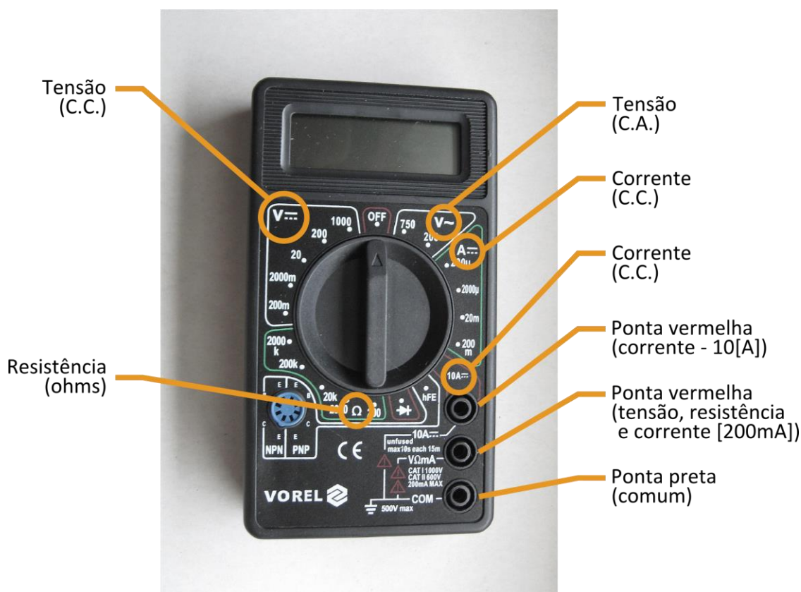
Fig. 4.2 Multímetro.
