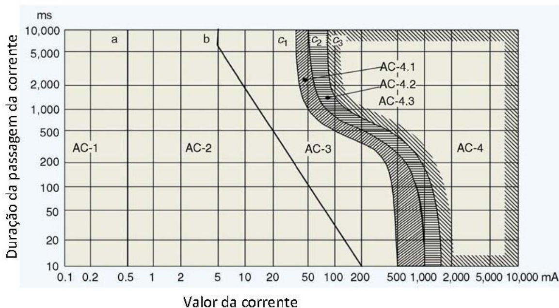
Fig. 3.6 Zonas de efeito da corrente alternada (15-100 Hz) em uma pessoa, cuja corrente atravessa seu corpo entrando pela mão esquerda e saindo pelo pé.
