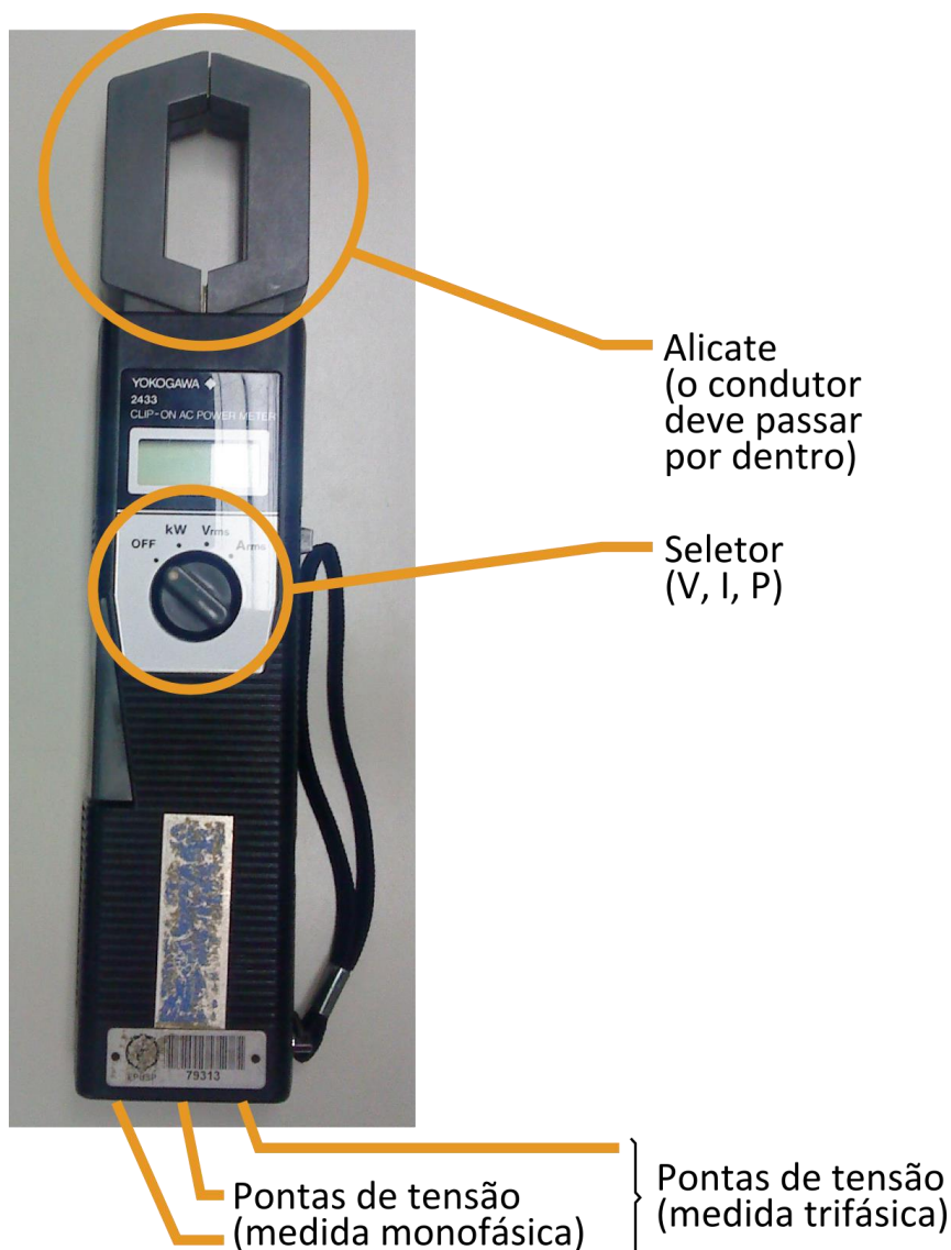
Fig. 4.2 Wattímetro de alicate.
