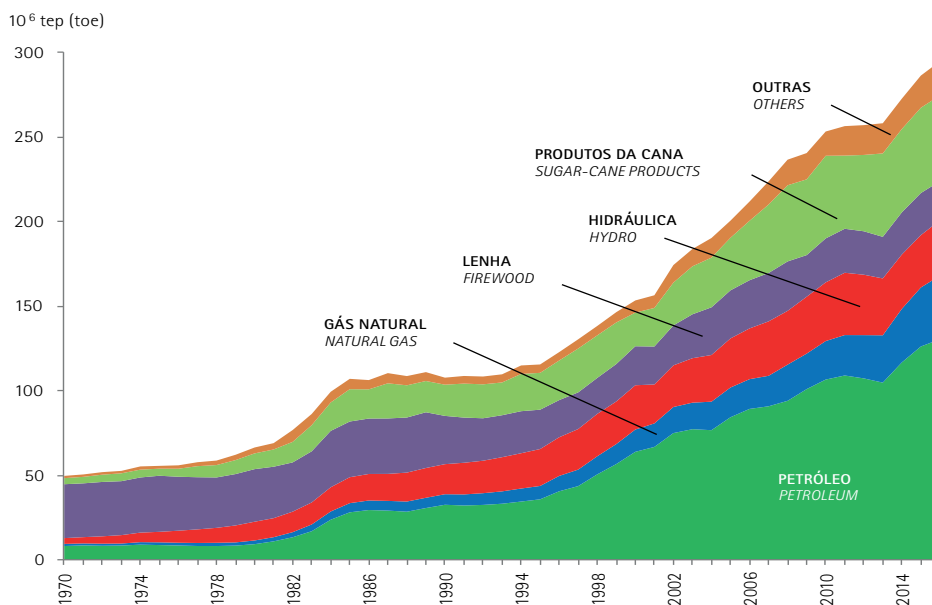
Gráfico 1.2.a – Produção de Energia Primária
