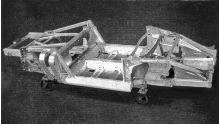
Fig. 18.1-27 Final 360 Modena spaceframe.
