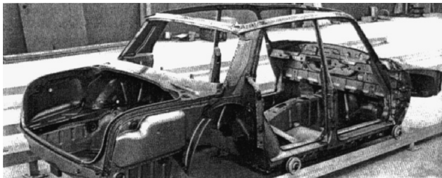
Fig. 18.1-24 Rover P6 spaceframe.
