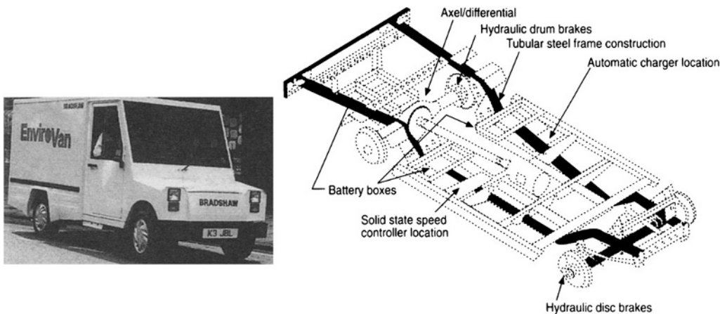
Fig. 6.1-22 Bradshaw Envirovan.
