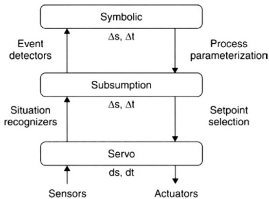
Fig. 14.2-6 SSS architecture (Connell).
