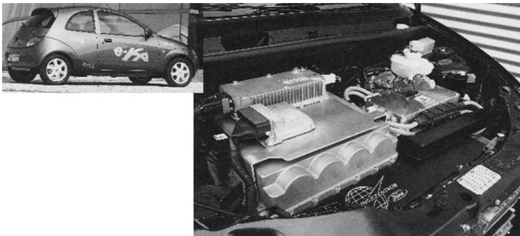
Fig. 6.1-17 Ford e-Ka.
