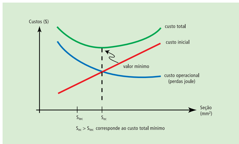
Gráfico 1: Custo inicial e custo operacional dos cabos em função da seção nominal.
