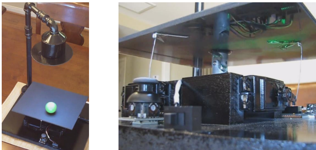
Figura 1 – Sistema de equilíbrio bola e prato, detalhe da atuação com dois servo motores.
