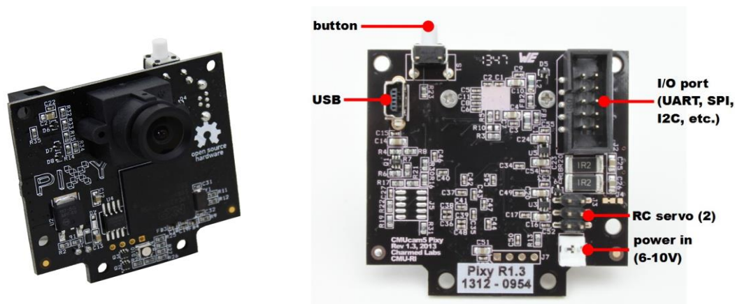
Figura 3 – PixyCam e parte traseira com conectores.
