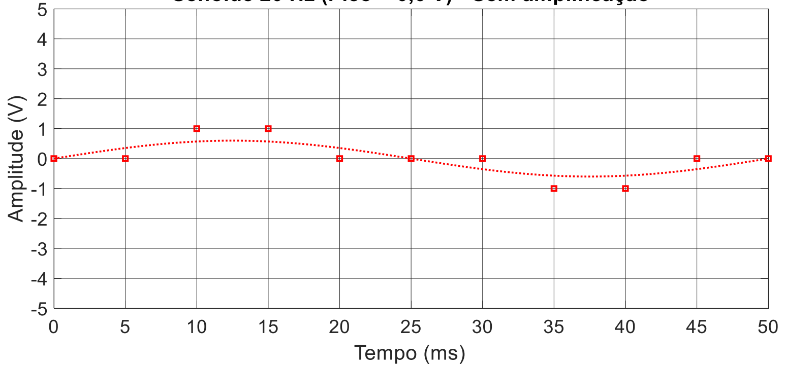
Senoide 20 Hz (Pico = 0,6 V) - Sem amplificação
