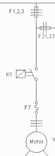
Diagrama de Unifilar
