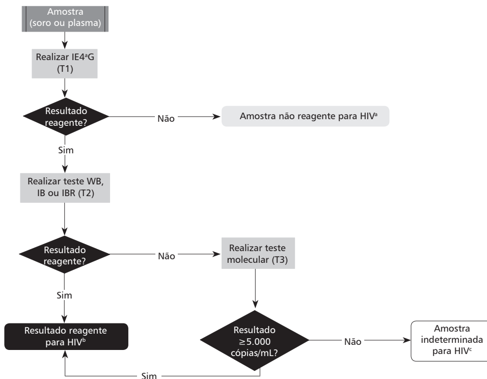
Figura 8 – Fluxograma 6: Imunoensaio de 4ª geração (IE4ªG) e western blot (WB), imunoblot (IB) ou imoblot rápido (IBR) como teste complementar
