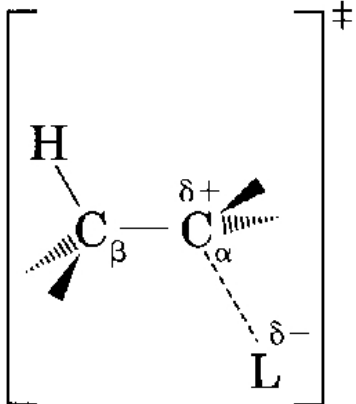
E1
