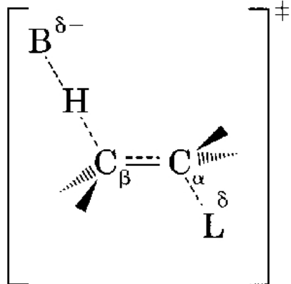
E2
