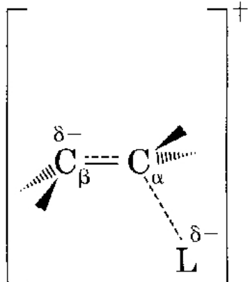
E1cb
