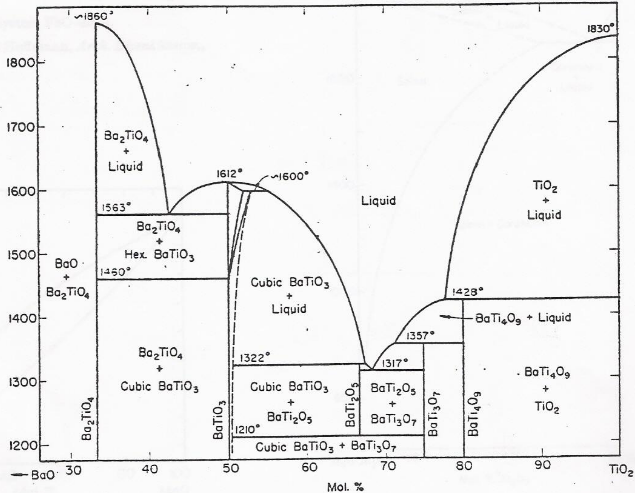
FIG. 213.—System BaO-TiO 2 .
