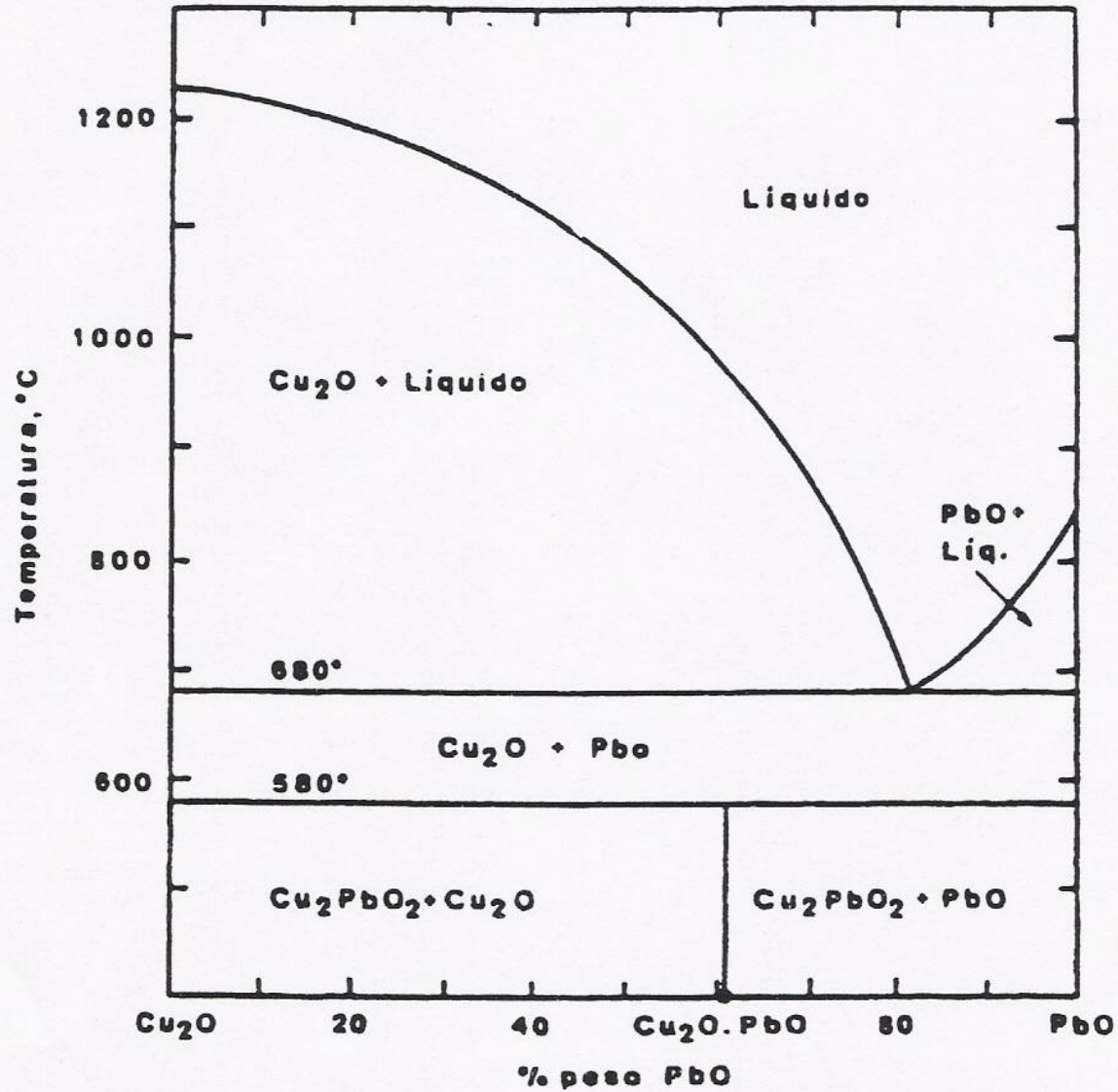
Figura 12: Diagrama de fases do sistema \text{Cu}_2\text{O} - \text{PbO} .
