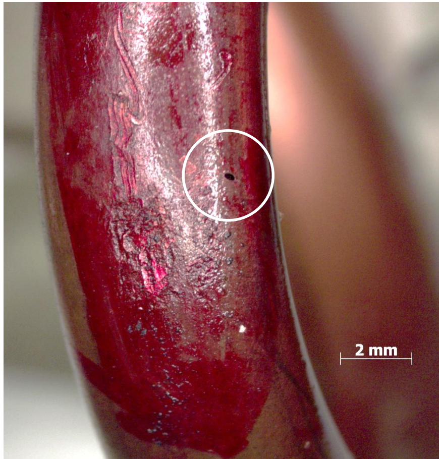
Figura 2 – Local em que foi encontrado furo na parede da serpentina de refrigeração.
