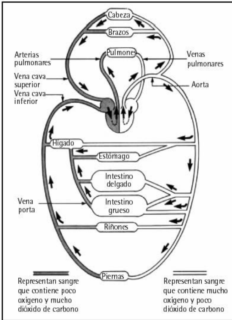
Figura 7. Esquema de la circulación de la sangre (Wheeler, 1981)
