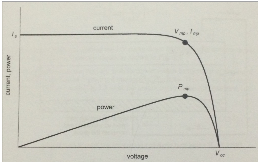
Foto 1: Curva típica do comportamento da célula
