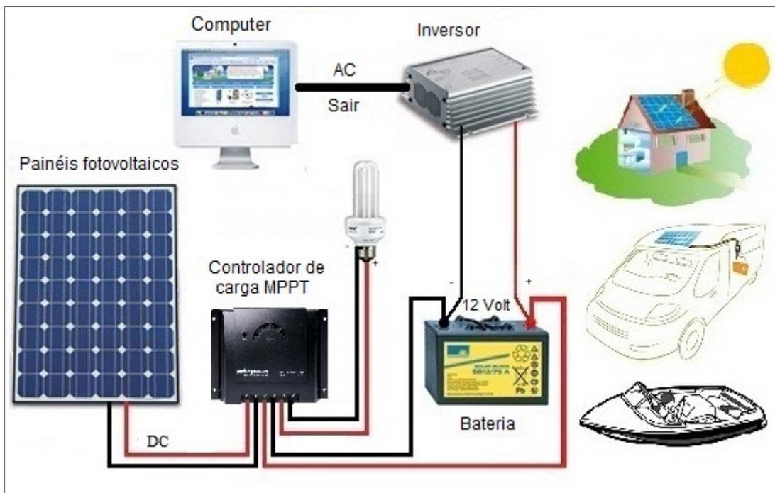
Esquema 1 – Diagrama elétrico fotovoltaico sistema on grid
